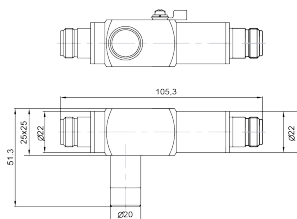
PRC350-N/FF
